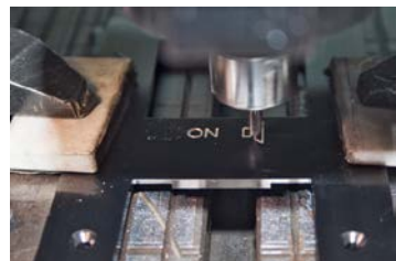
RECHTS: Sogenannte Wechselschalter aus Messing warten auf ihre Weiterverarbeitung. UNTEN: Anfang der 90er-Jahre wurden vor allem Holzmodelle produziert, die auch heute noch zur Kollektion gehören. Ab 2008 erfolgte die Spezialisierung auf Messing
